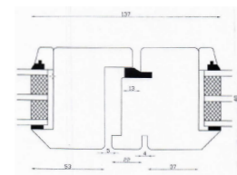
Detalje 62 1:5
