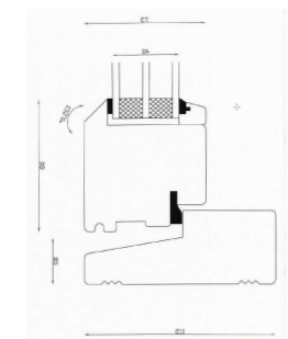
Detalje 213 1:5
