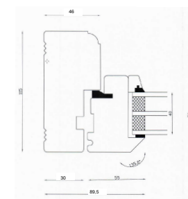
Detalje 55 1:5
