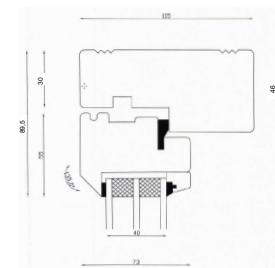
Detalje 54 1:5
